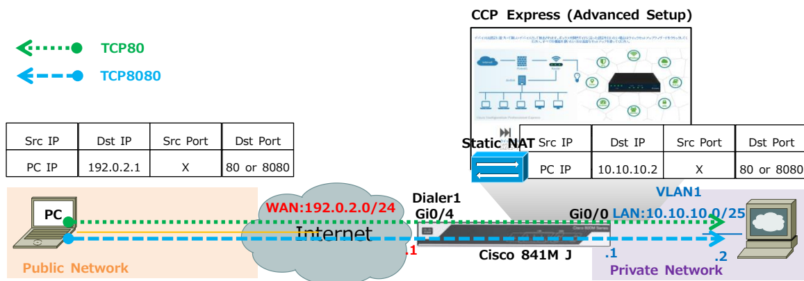
図 2 スタティック NAT の設定で構成するシステム
